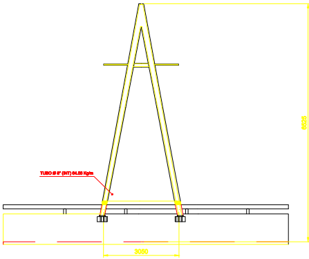
VISTA LATERAL
