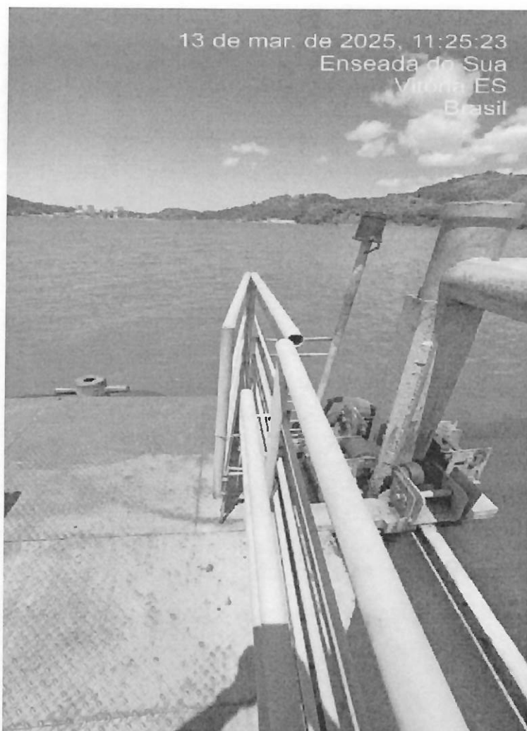
Figura 9 – Encontrado guarda corpo quebrado e passarela de embarque e desembarque com avarias ocasionadas por colisões de embarcações.
