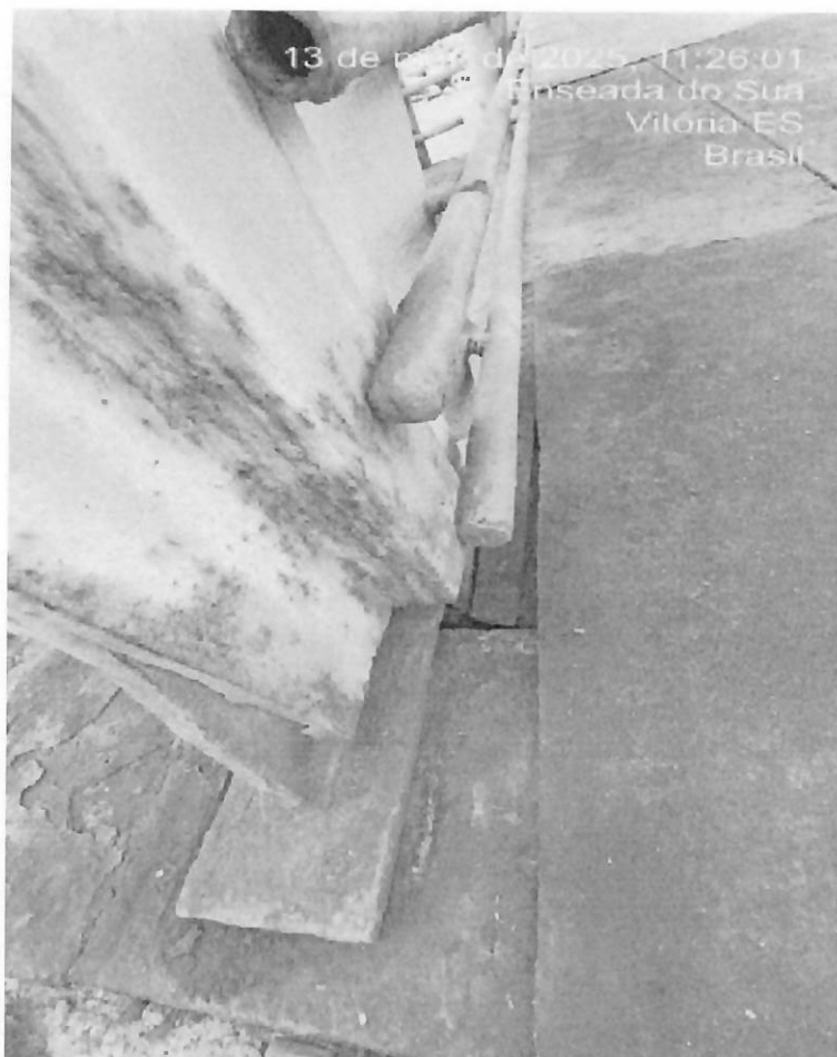
Figura 11 – Diferença de desnível prejudicando patola de apoio para içamento e manutenção.
