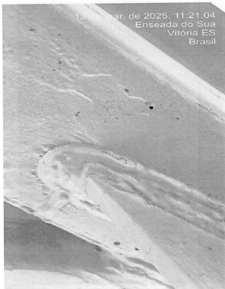
Figura 2 - Trinca no mesmo local da última ocorrência relacionada a transferência de torção do flutuante para a passarela – Entrada da bilheteria ao flutuante superior lado direito.
